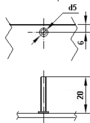
расположение шпильки относительно края монитора
