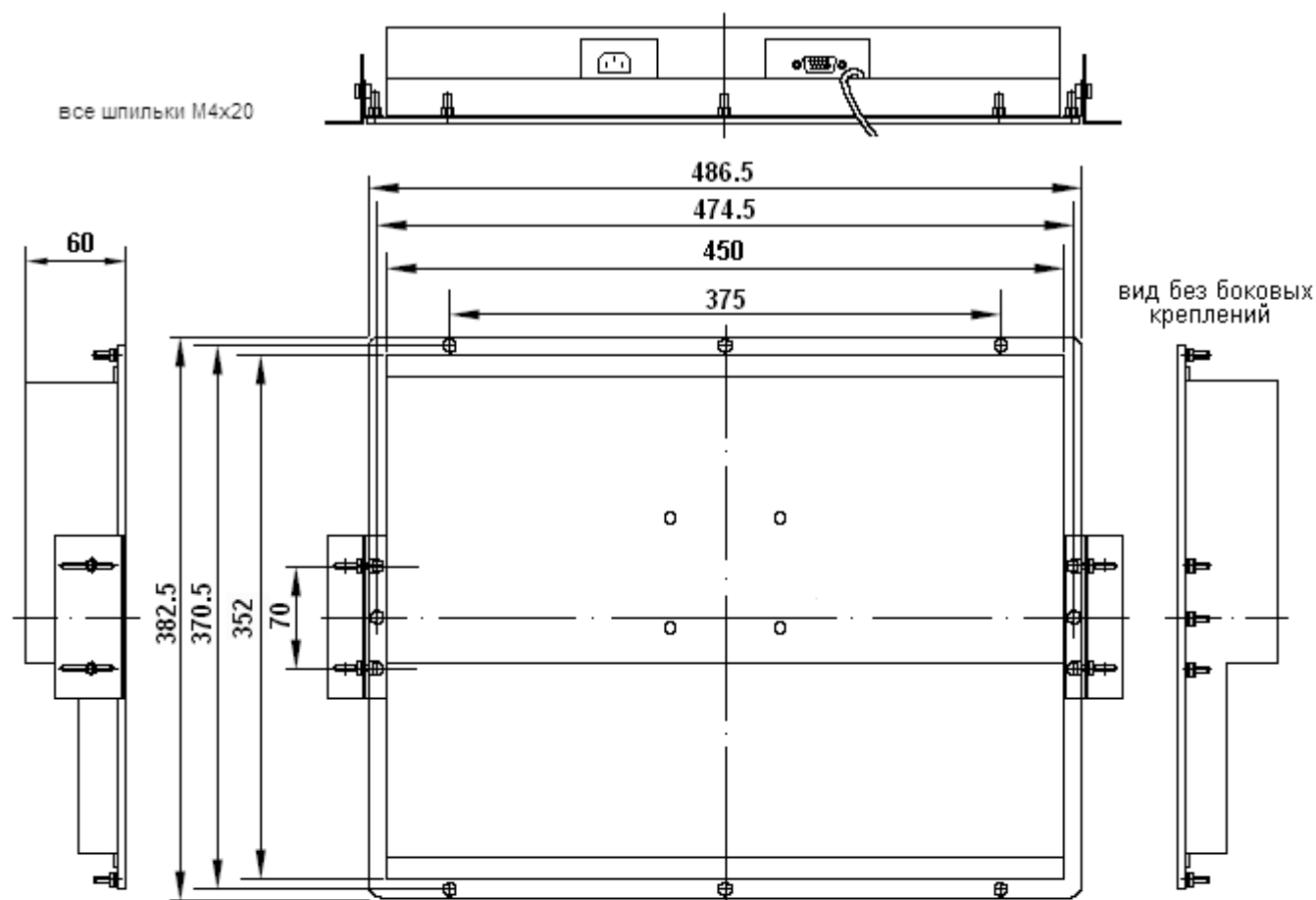
размер выреза в корпусе киоска для посадки монитора
